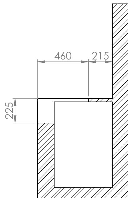
SEÇÃO C-C
